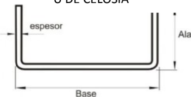
U DE CELOSLA
